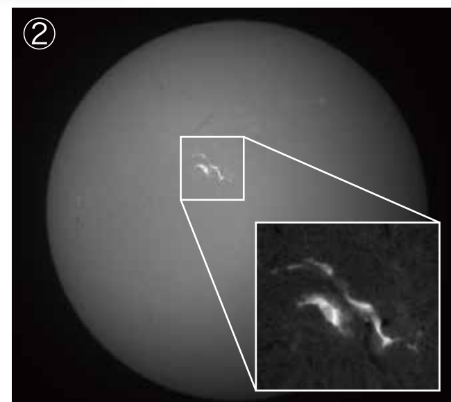
①太陽プロミネンス（2022年9月15日） ②中規模フレア（2021年11月2日） 別館：18cm屈折ザートリウス望遠鏡。晴天時には、リアルタイムの太陽画像を観察できます。
