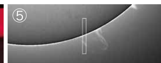
秒速数10kmで運動するプロミネ ンス（右図⑤）のスペクトル（左図④ ：H \alpha 線、左方向が短波長、右方向 が長波長）2022年7月2日 左図は太陽館、右図は別館で撮影
